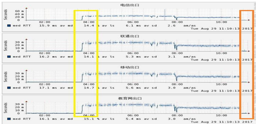
图 2 校园网出口监控显示 11 点左右恢复正常
