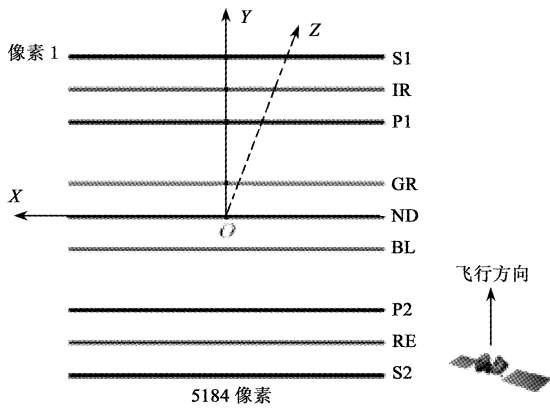
图 4 HRSC 相机线阵 CCD 排列 Fig. 4 HRSC Linear array camera
