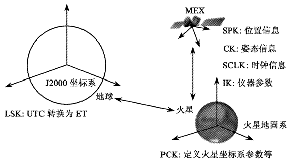
图 5 利用 SPICE 库获取 HRSC 外方位元素 Fig. 5 Obtaining EO using SPICE kernels
