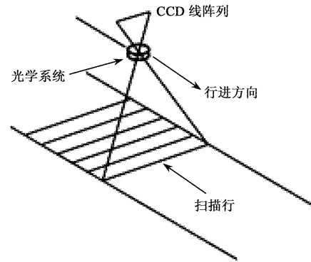
图 6 线阵 CCD 影像推扫式示意图 Fig. 6 Imaging principle of linear pushbroom imagery
