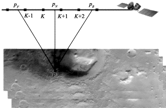
图 7 线阵传感器定向片模型
