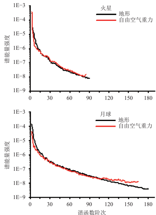
图1 月球与火星的重力异常频谱特性对比
