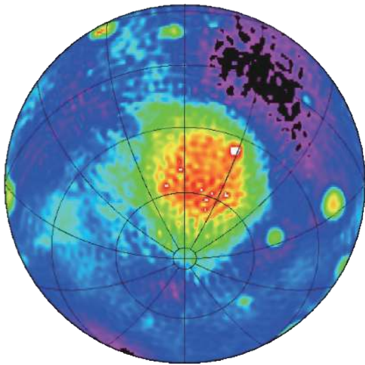
图 4 月球背面南极周边区域布格重力异常分布
