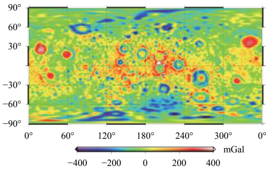
图2 月面上空10 km球面处月球重力场模型的全球重力异常分布 Fig. 2 Lunar gravity anomaly distribution of 10 km above lunar average surface sphere
