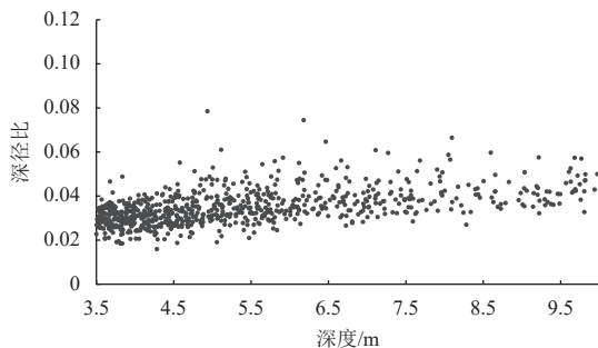
图10 深度大于3.5 m的撞击坑深径比情况
