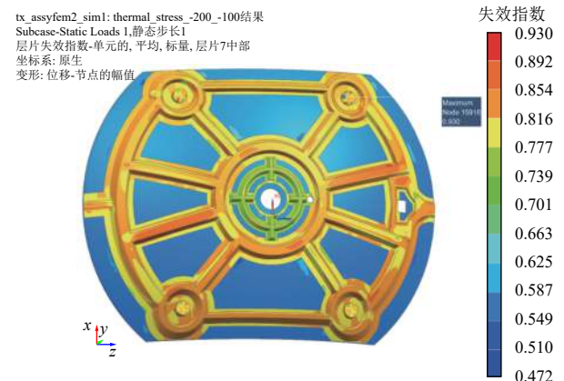
图 5 -200℃低温工况反射面部件层片的失效指数云图 Fig. 5 Failure index map of reflector components at -200℃
